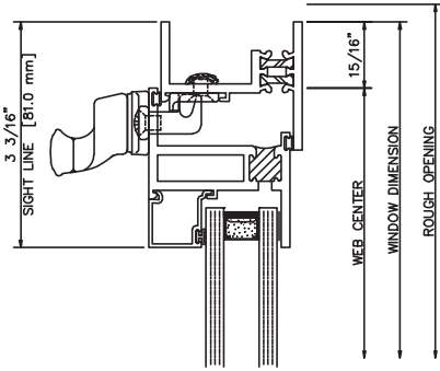
421 RIGHT JAMB
