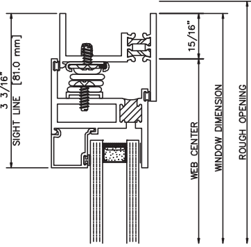
403 RIGHT JAMB
