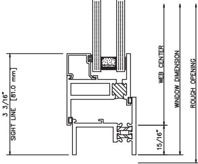
420 LEFT JAMB
