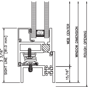
402 LEFT JAMB
