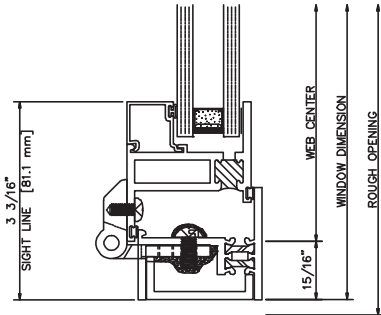
424 LEFT JAMB
