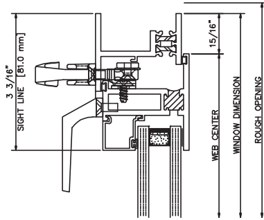
413 RIGHT JAMB
