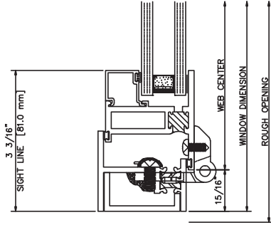
412 LEFT JAMB
