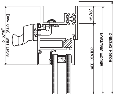
421 RIGHT JAMB
